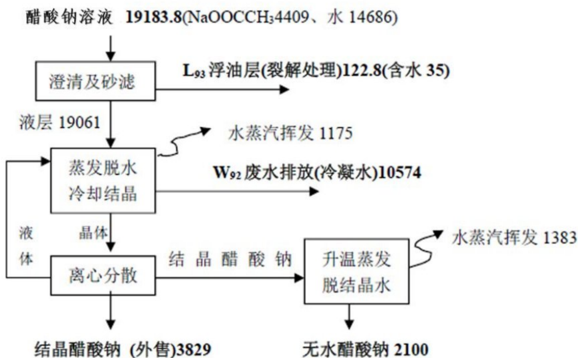
图3.3-3 醋酸钠回收利用装置工艺流程图
