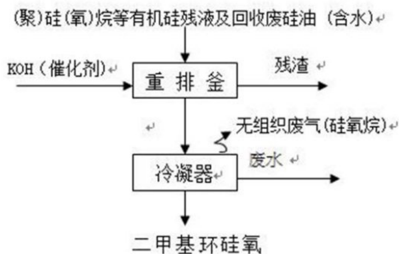
图3.3-4 硅油重排回收利用工艺流程图
