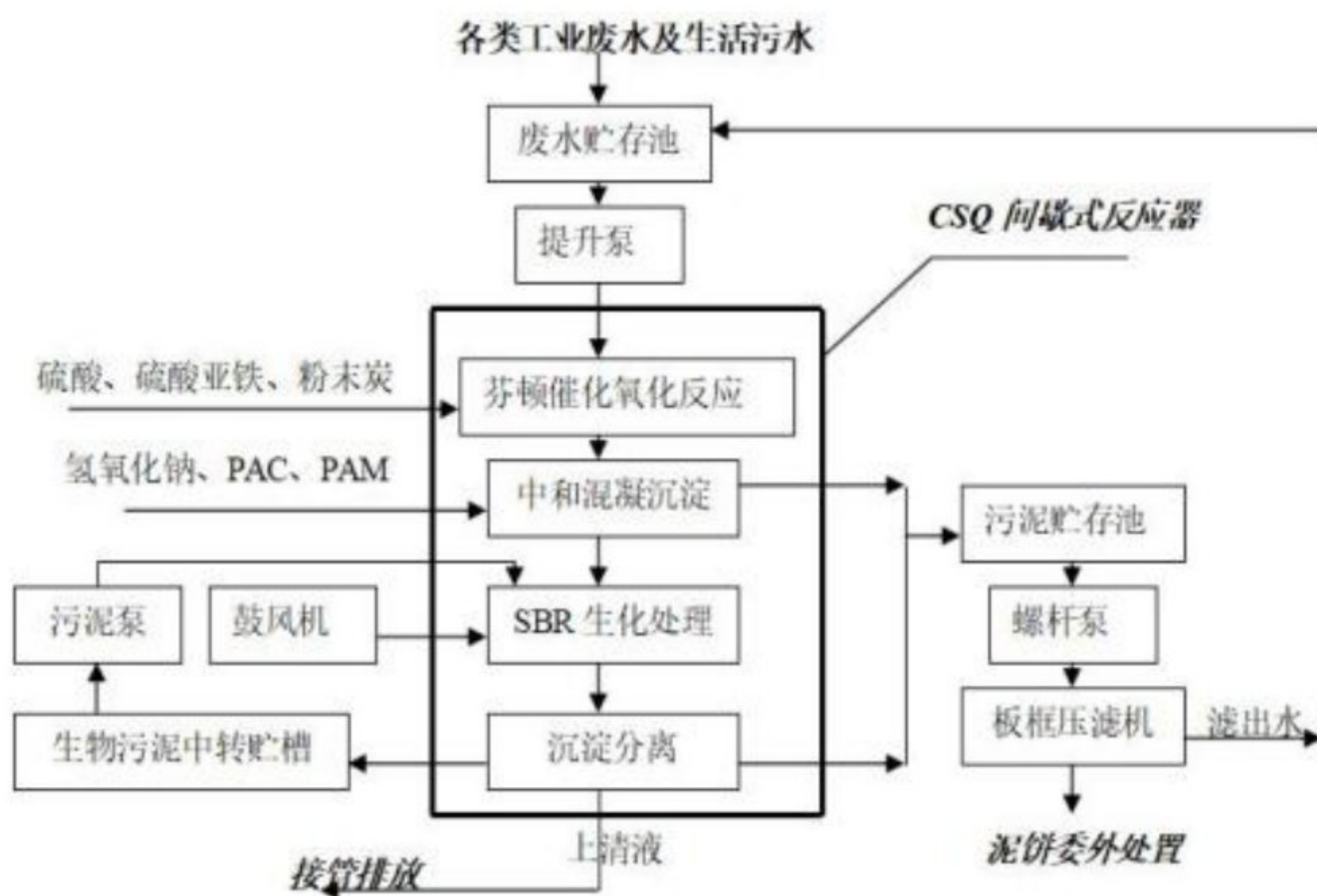
图3.5-2 废水处理工艺流程图
