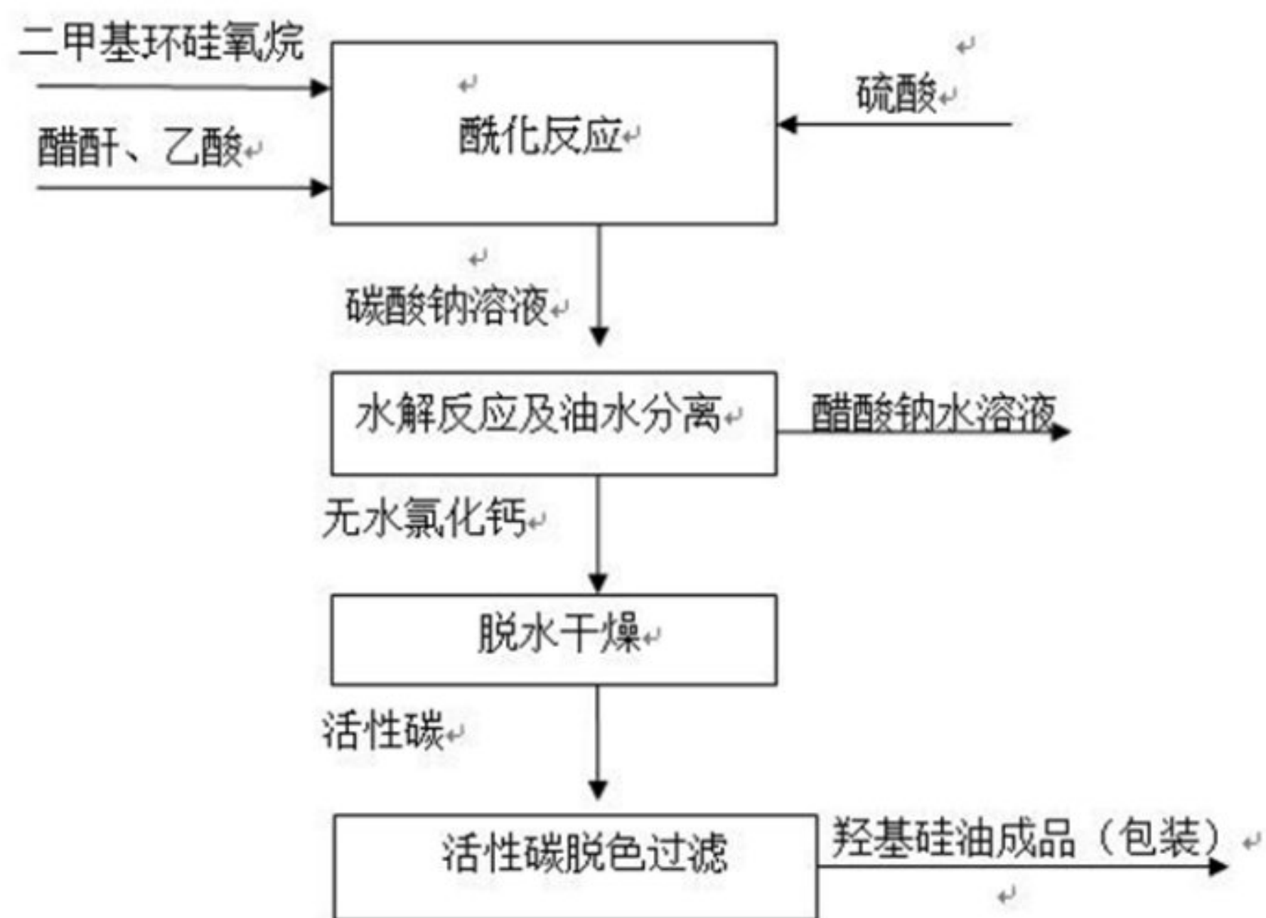
图3.3-2 羟基硅油工艺流程、主要产污环节图
